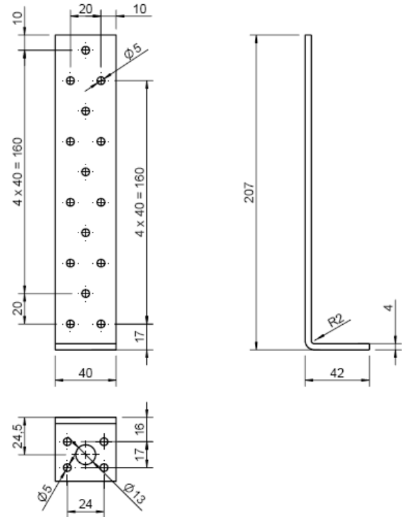
Bild A.4 Maße des Betonflachstahllanker 40 x 200 x 4,00
