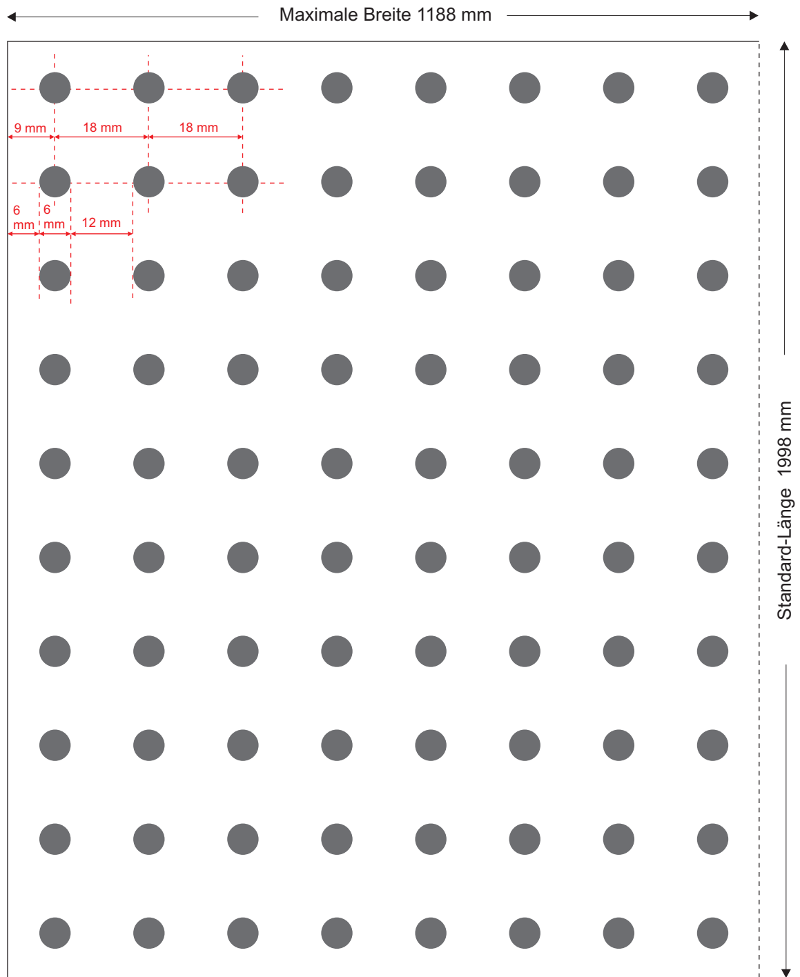
Plattenausschnitt, Maßstab 1:1
