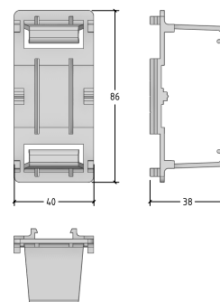
Kreuzverbinder TWIXT 33-65 mm
