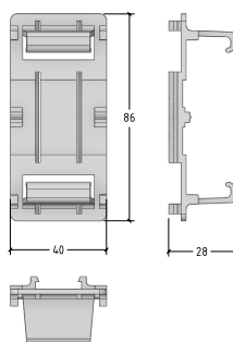
Kreuzverbinder FLAT 23-32 mm
