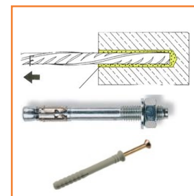
Wandbefestigung (bauseits)
