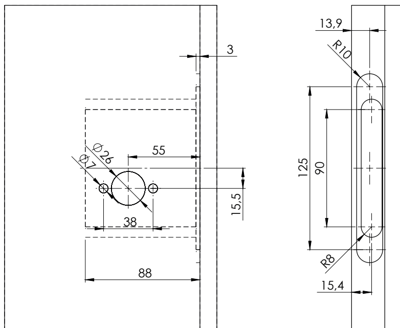
Bohrung für Türbeschlag Drilling for door fitting
