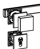
Wechselgarnitur PZ mit Knopf Square
