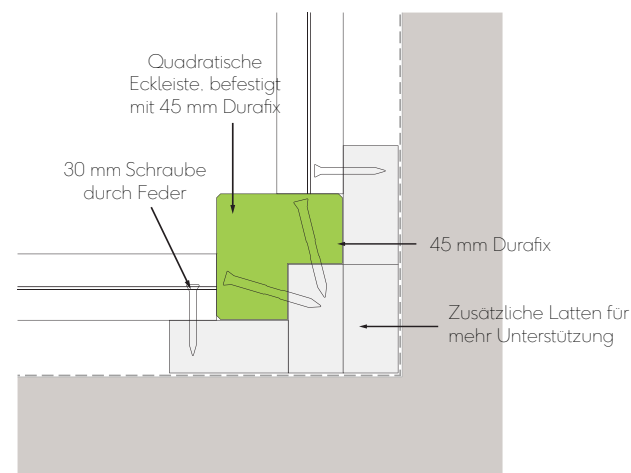
Abb. 7 - Details der Innenecke
