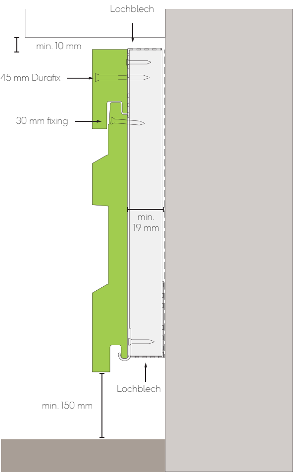
Abb. 1 - Details der oberen und unteren Verkleidung
