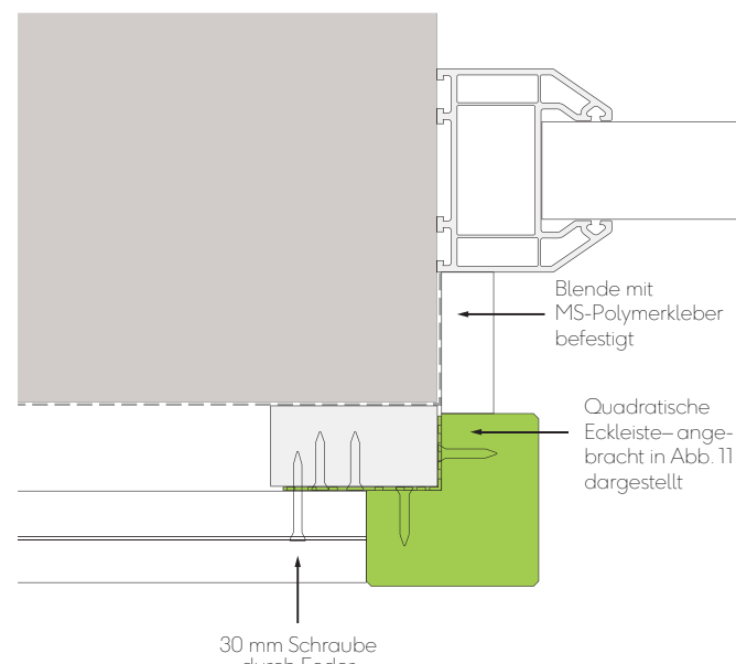
Abb. 12 - Fenster-/Türpfosten mit Eckprofil
