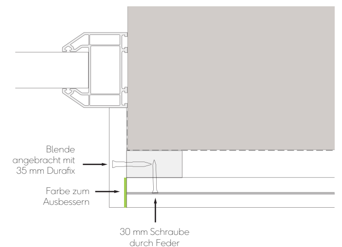
Abb. 16 - Fenster-/Türpfosten mit Blenden
