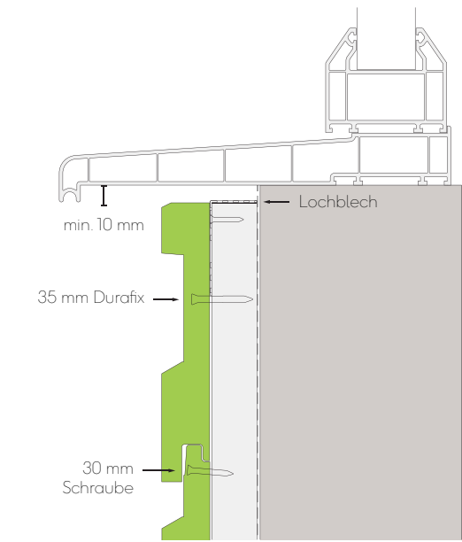
Abb. 3 - Detail Fenster/Türschwelle
