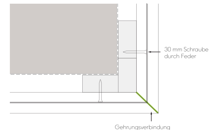
Abb. 10 - Details der auf Gehrung geschnittenen Außenecke
