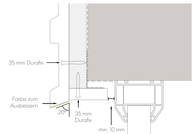
Abb. 14 - Fenster-/Türsturz mit Schrägschnitt
