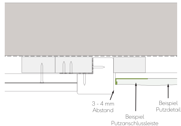
Abb. 20 - Eckprofil stößt an den Putz an
