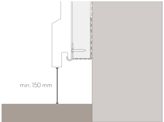
Abb. 4 - Einbaudetail über Bodenhöhe
