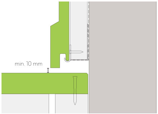
Abb. 5 - Einbaudetails über Terrassendiele
