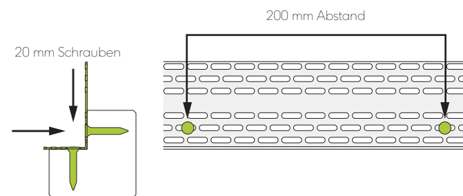
Abb. 11 - Verwendung von Lochblechen an externen Eckprofilen
