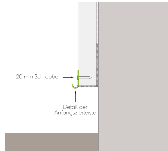
Abb. 17b - Detail der Anfangszierleiste
