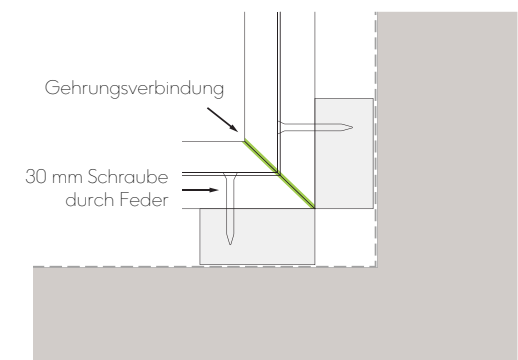
Abb. 9 - Details der auf Gehrung geschnittenen Innenecke
