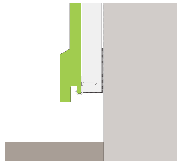
Abb. 18 - Erste Paneelmontage
