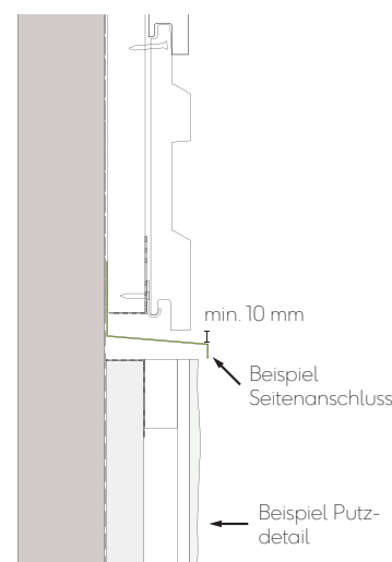
Abb. 22 - Anbringen von Verkleidungen über Putz
