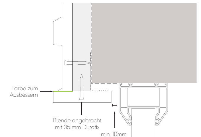
Abb. 15 - Fenster-/Türsturz mit Blende
