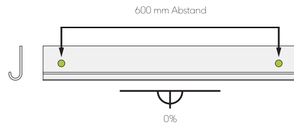
Abb. 17a - Anfangszierleiste montieren
