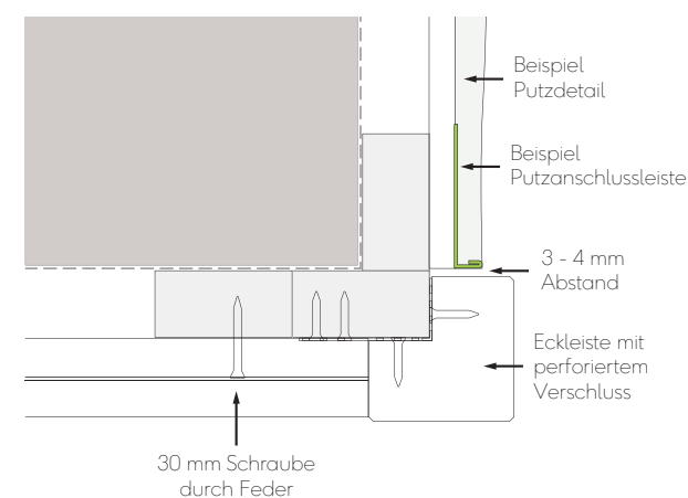
Abb. 21 - Eckprofil stößt an der Außenecke an den Putz an
